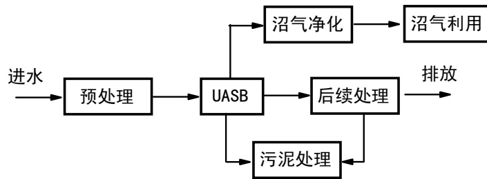
图 1 工艺流程图
