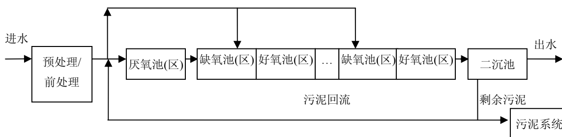
图 A.5 MAO 工艺流程图
