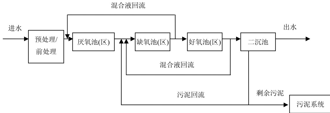
图 A.1 UCT 工艺流程图
