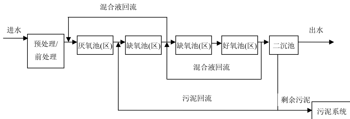
图 A.2 MUCT 工艺流程图
