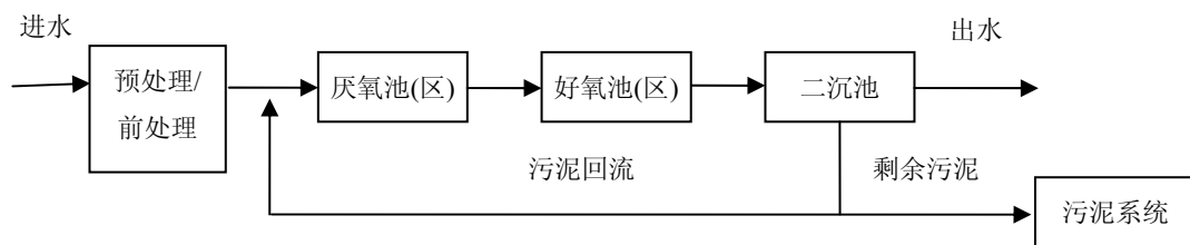
图 1 厌氧好氧工艺流程
