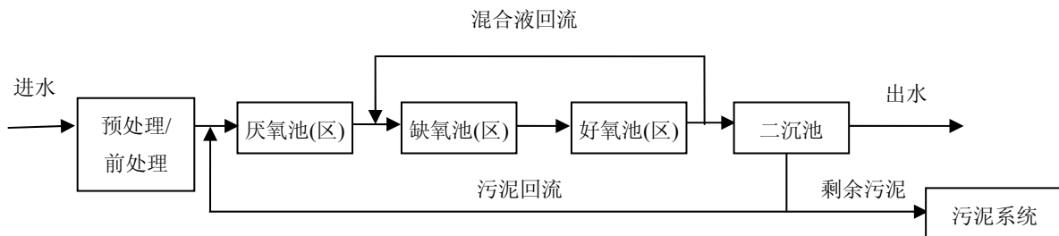
图 3 厌氧缺氧好氧工艺流程图
