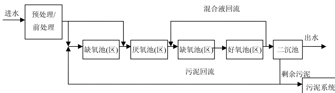
图 A.3 JHB 工艺流程图
