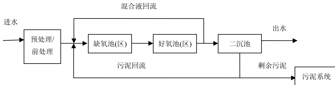
图 2 缺氧好氧工艺流程
