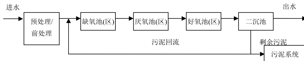
图 A.4 RAAO 工艺流程图
